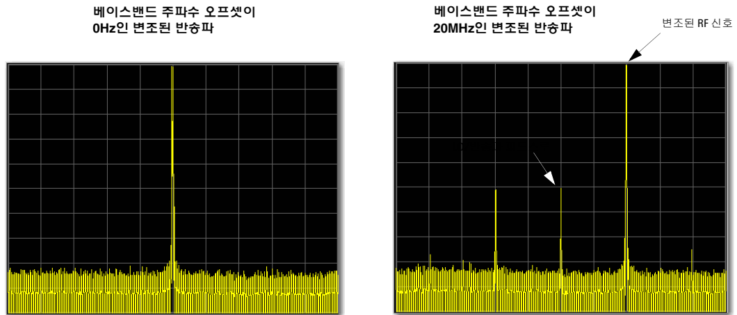
100MHz 범위로 설정된 스펙트럼 분석기
