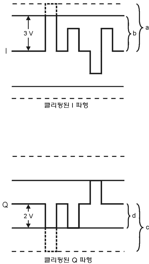
그림 8-11 사각 클리핑
