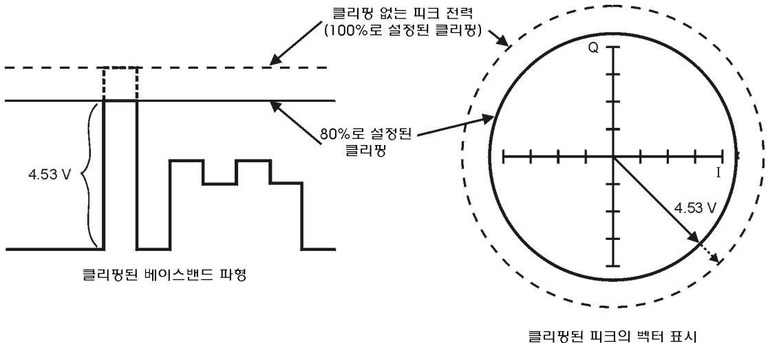
그림 8-10 원형 클리핑
