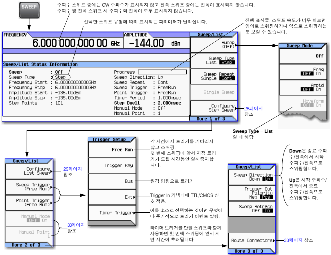
그림 3-2 스위프 Softkeys
